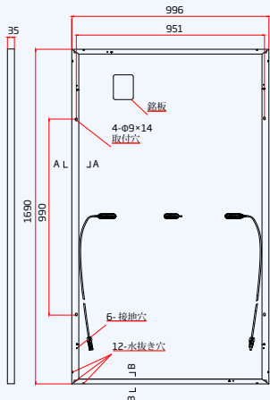
裏面図
